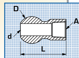
Rotule d'adaptation longue Type OB
